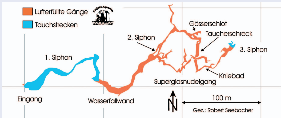
Abb. 2: Höhlenverlaufsplan der Schwarzen Lacke im Grundriss.
